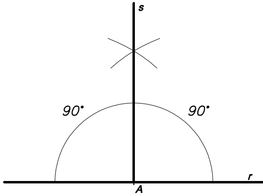
1- CONSTRUCCIÓ D'UN ANGLE DE 90°
