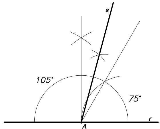
6- CONSTRUCCIÓ D'UN ANGLE DE 75° I 105°
