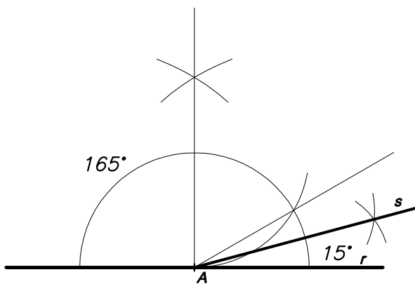
5- CONSTRUCCIÓ D'UN ANGLE DE 15° I 165°
