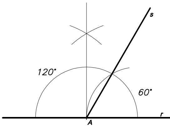
3- CONSTRUCCIÓ D'UN ANGLE DE 60° I 120°
