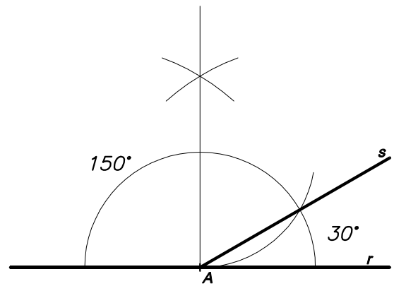
4- CONSTRUCCIÓ D'UN ANGLE DE 30° I 150°
