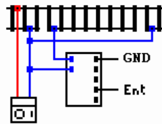
Detector presencia
