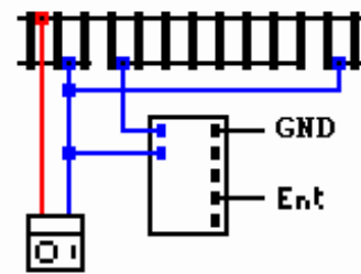
Detector presencia
